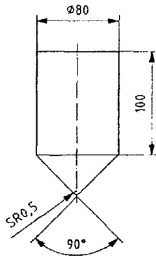
Hình 5: Đầu thử hình côn
