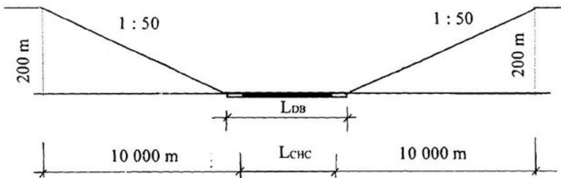
Hình 8a-PLI: Mặt cắt dọc dài tính không đầu đường sân bay
