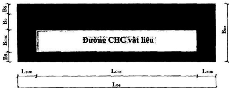
Hình 1-PLI: Sơ đồ dài bay sân bay quân sự
