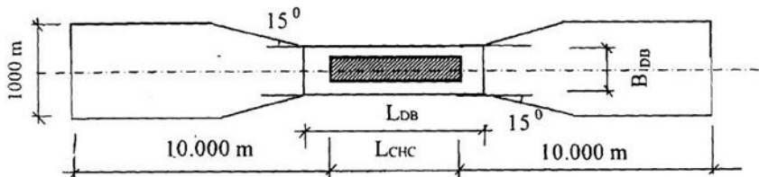
Hình 8b-PLI: Mặt bằng dài tính không đầu đường sân bay
