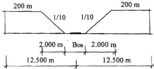
Hình 9-PLI: Kích thước dài tĩnh không sườn đường sân bay
