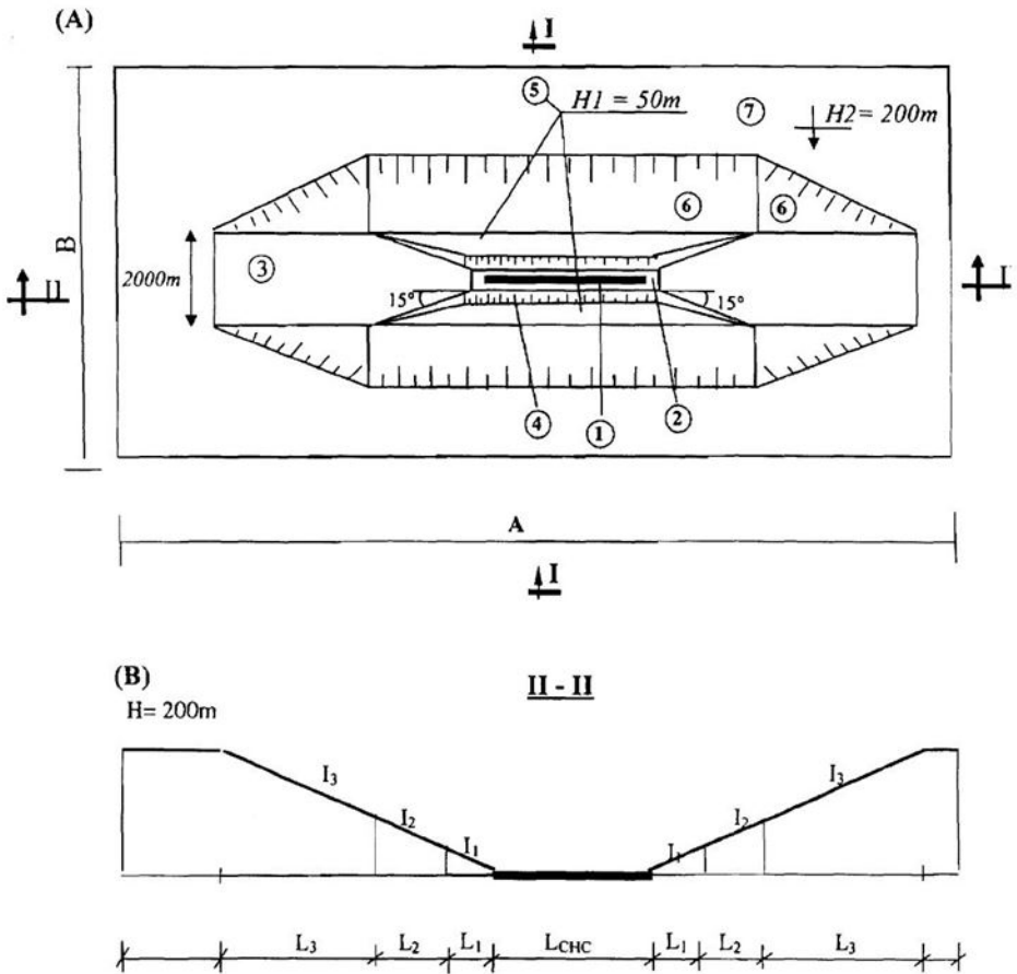
Hình 4a-PLI: Mặt bằng dài phụ cận đầu sân bay quân sự.
