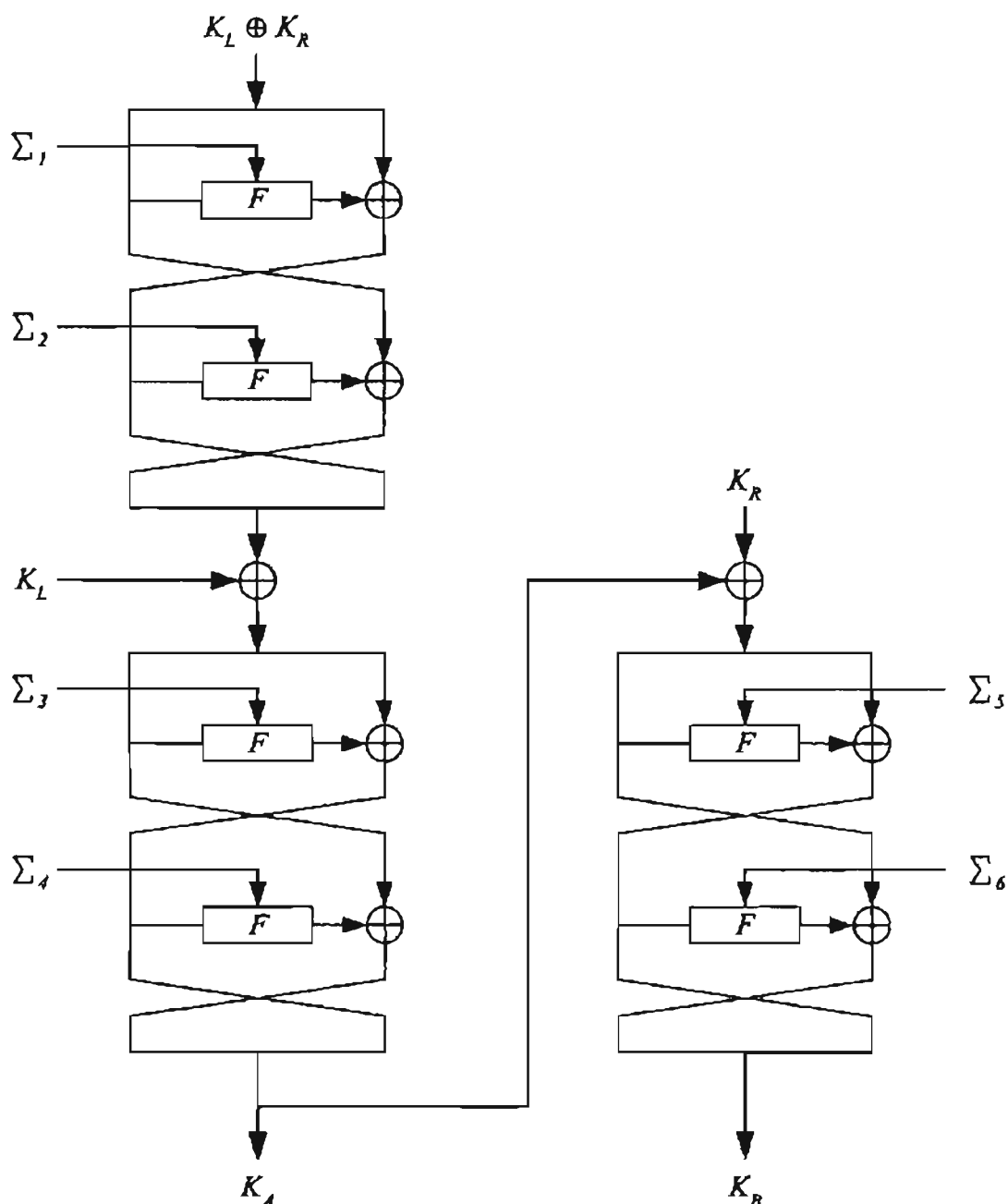
Hình 7: Phần chính của lược đồ khóa
