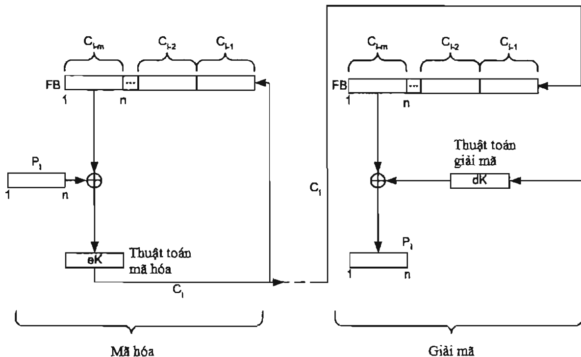
Hình 9: Chế độ xích liên kết khối mã
